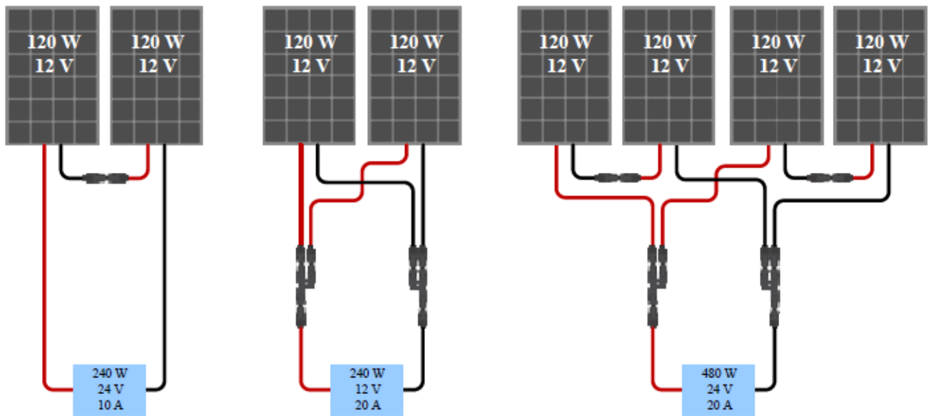
串聯、並聯及串並聯太陽能陣列範例。
