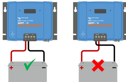
正確與不正確（反接）電瓶極性範例
