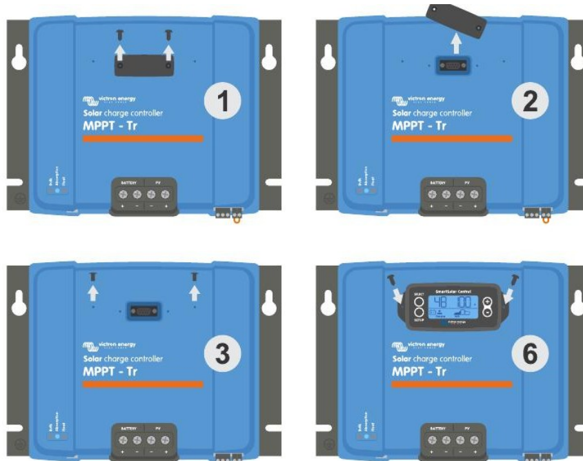
如何及在何處連接 SmartSolar Control 顯示器
