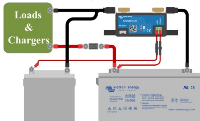
電瓶監視器搭配選項第二電瓶監視功能。
