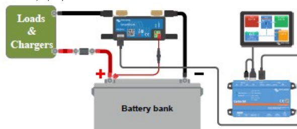
電瓶監視器連接至 Cerbo GX 及 GX Touch 螢幕。
