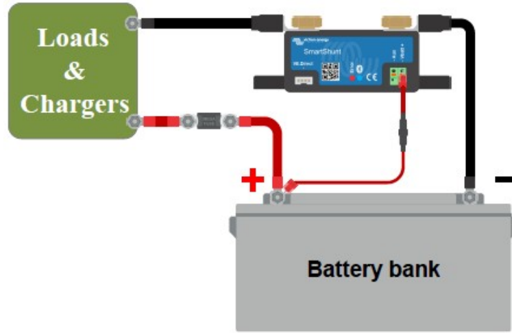
基本電瓶監視器安裝。
