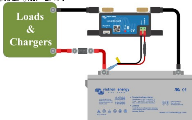
電瓶監視器搭配選項溫度感測功能。
