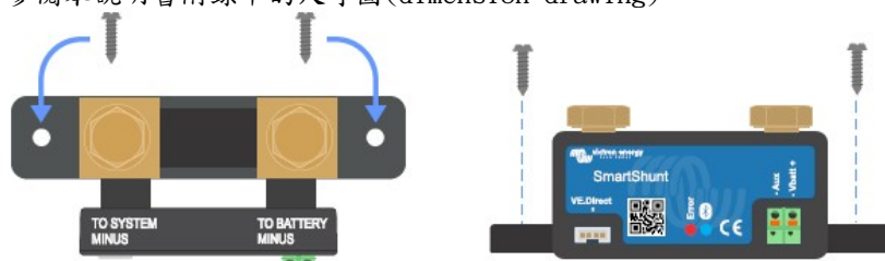
SmartShunt 俯視圖（標示安裝孔）及側視圖（標示安裝方式）。
