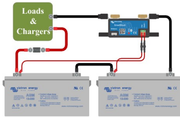
電瓶監視器搭配選項中點監視功能。
