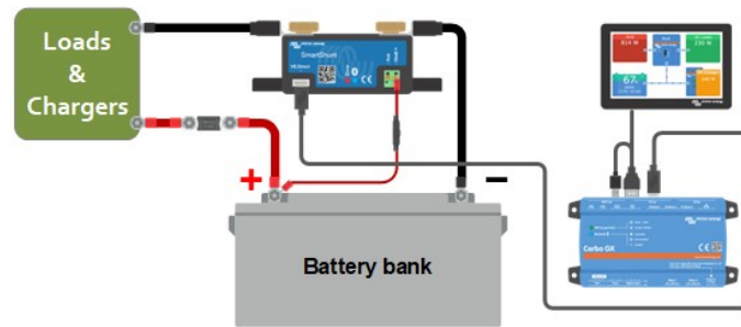
電瓶監視器連接至 GX 裝置的範例。
