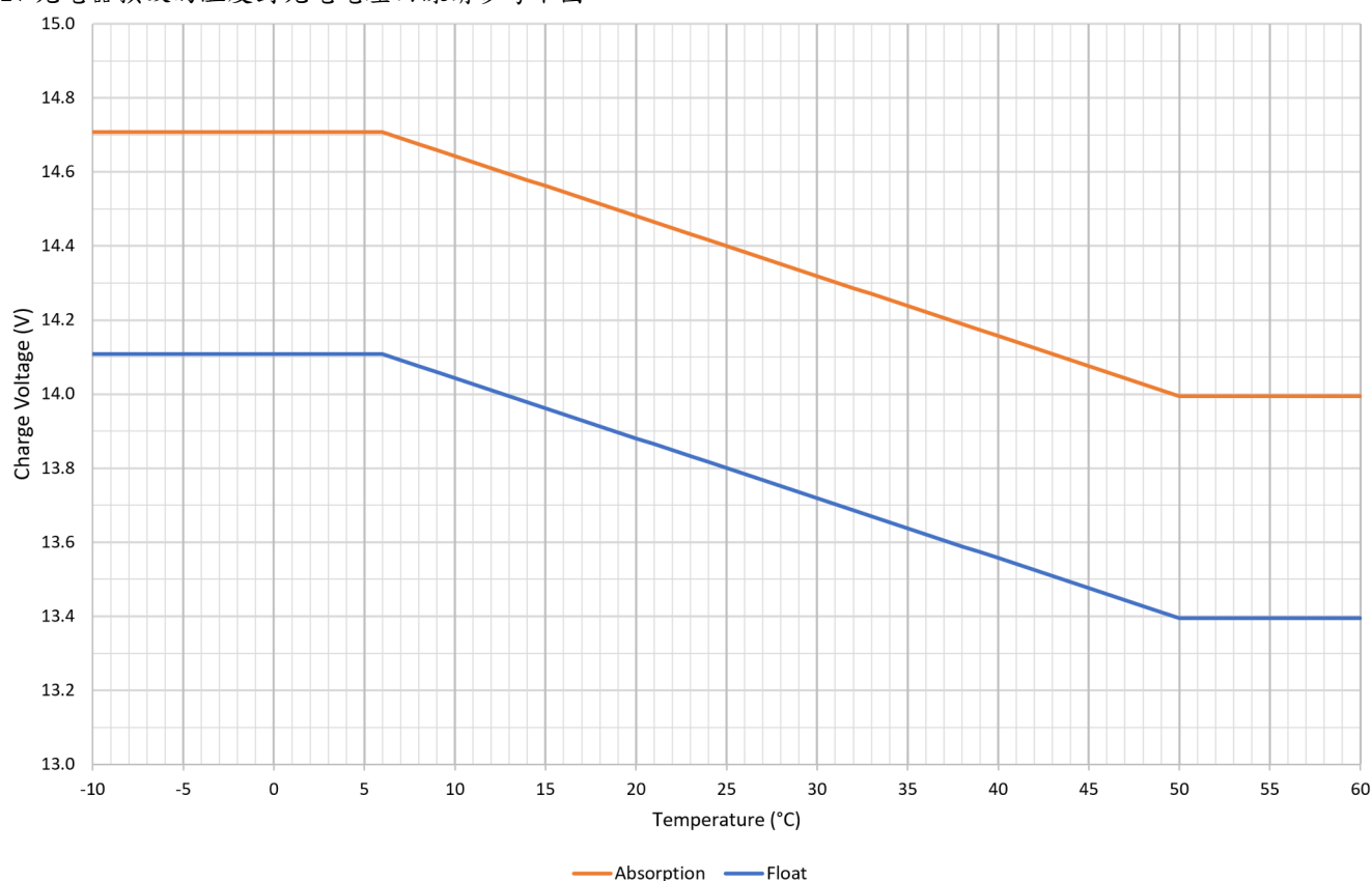
圖：12V 充電器溫度補償曲線
