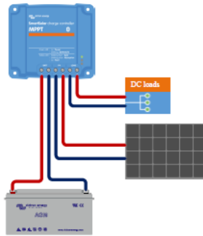
DC 負載連接至負載輸出的太陽能充電系統
