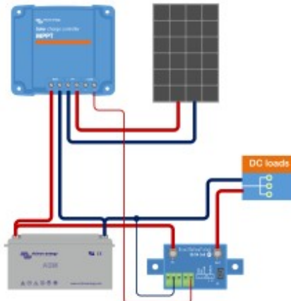
DC 負載透過電瓶保護器直接連接至電瓶、並由負載輸出控制的太陽能充電系統
