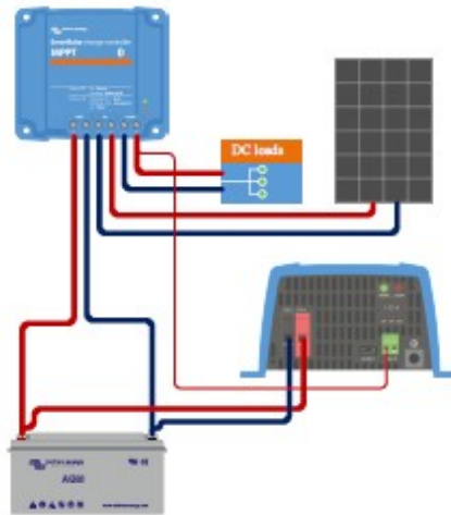
變流器直接連接至電瓶、並由負載輸出控制的太陽能充電系統
