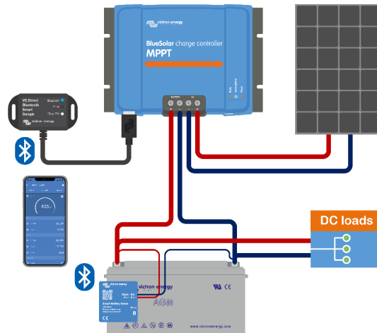
Smart Battery Sense 與太陽能充電器組成 VE.Smart 網路範例。
