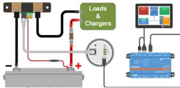
電瓶監視器連接至 GX 裝置的範例。
