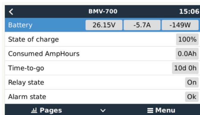
GX 裝置顯示的電瓶監視器資訊。
