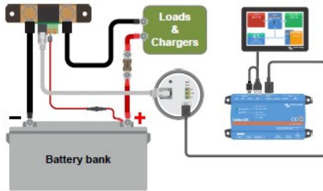
電瓶監視器連接至 Cerbo GX 及 GX Touch 螢幕。
