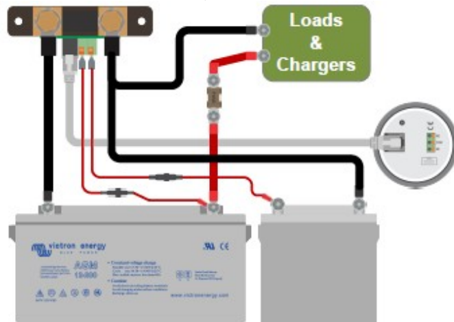
具第二個電瓶選項監視功能的電瓶監視器。
