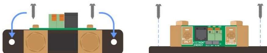
分流器上視圖（標示安裝孔）及側視圖（標示安裝方式）。
