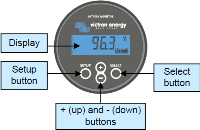
BMV 錶頭的顯示幕及按鍵。
