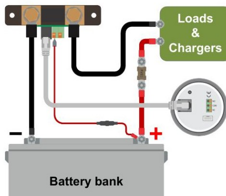
基本電瓶監視器安裝。
