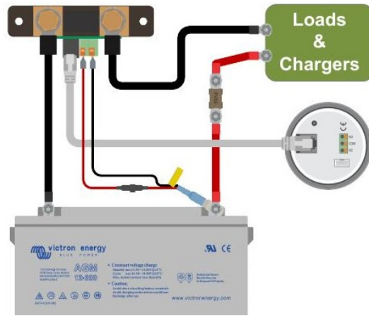
具溫度選項感測功能的電瓶監視器。
