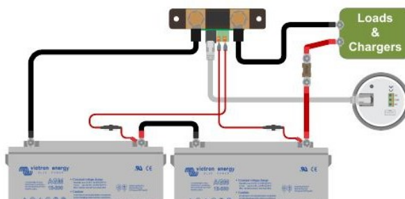
具中點選項監視功能的電瓶監視器。
