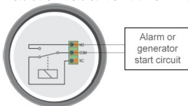
電瓶監視器內部線路圖，圖中繼電器處於未送電狀態，並連接至外部警報或發電機啟動迴路。
